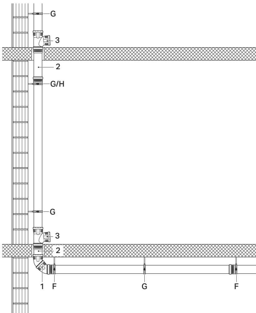
Abbildung 18: Umlenkung 2 x Bogen 45° mit Geberit Silent-Pro
