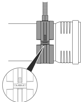
Abbildung 6: Festschelle bei der Steckmuffe
