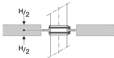
Abbildung 13: Einbautiefe Geberit Mauerkragen
