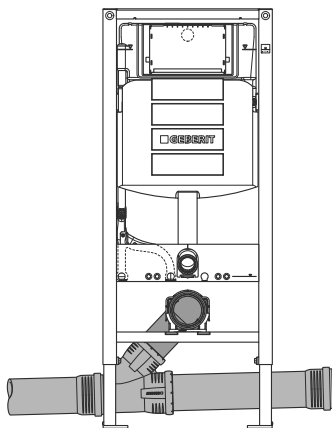
Abbildung 21: Anschlussmöglichkeit von WC-Abgang. WC-Abgangsbogen mit Außendurchmesser 90 und 110 mm können direkt in Geberit Silent-Pro Steckmuffen eingesteckt werden.
