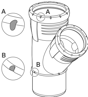
Abbildung 1: Positioniernocken
