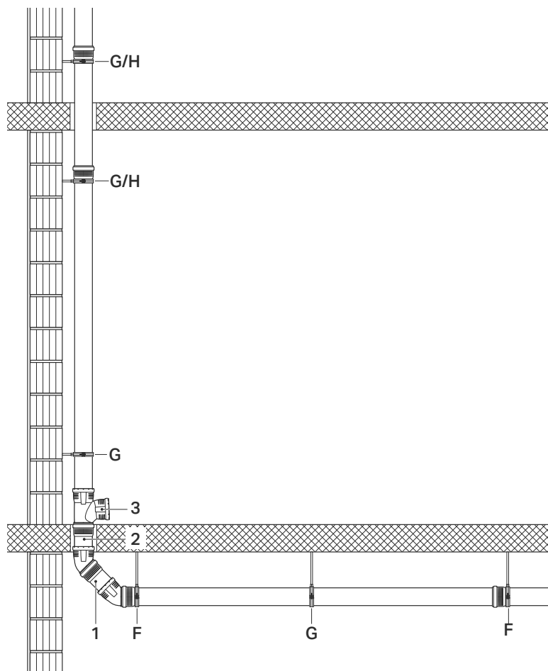
Abbildung 16: Umlenkung 2 x Bogen 45° und Beruhigungsstrecke mit Geberit Silent-Pro
