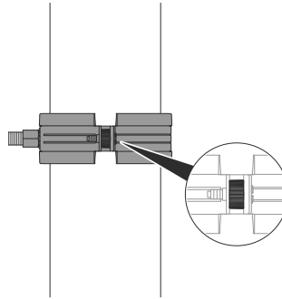
Abbildung 5: Gleitschelle mit Abstandhalter an der vertikalen Leitung
