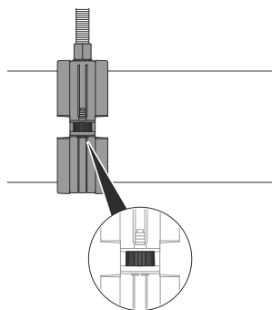
Abbildung 7: Zusätzliche Gleitschelle bei der horizontalen Leitungsführung
