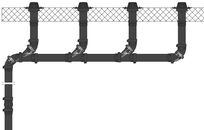
Abbildung 10: Innenliegende Regenwasserleitung Geberit Silent-Pro in Verbindung mit der Geberit Haltekralle
