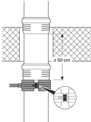
Abbildung 4: Positionierung der Gleitschelle mit zusätzlichem Rohr
