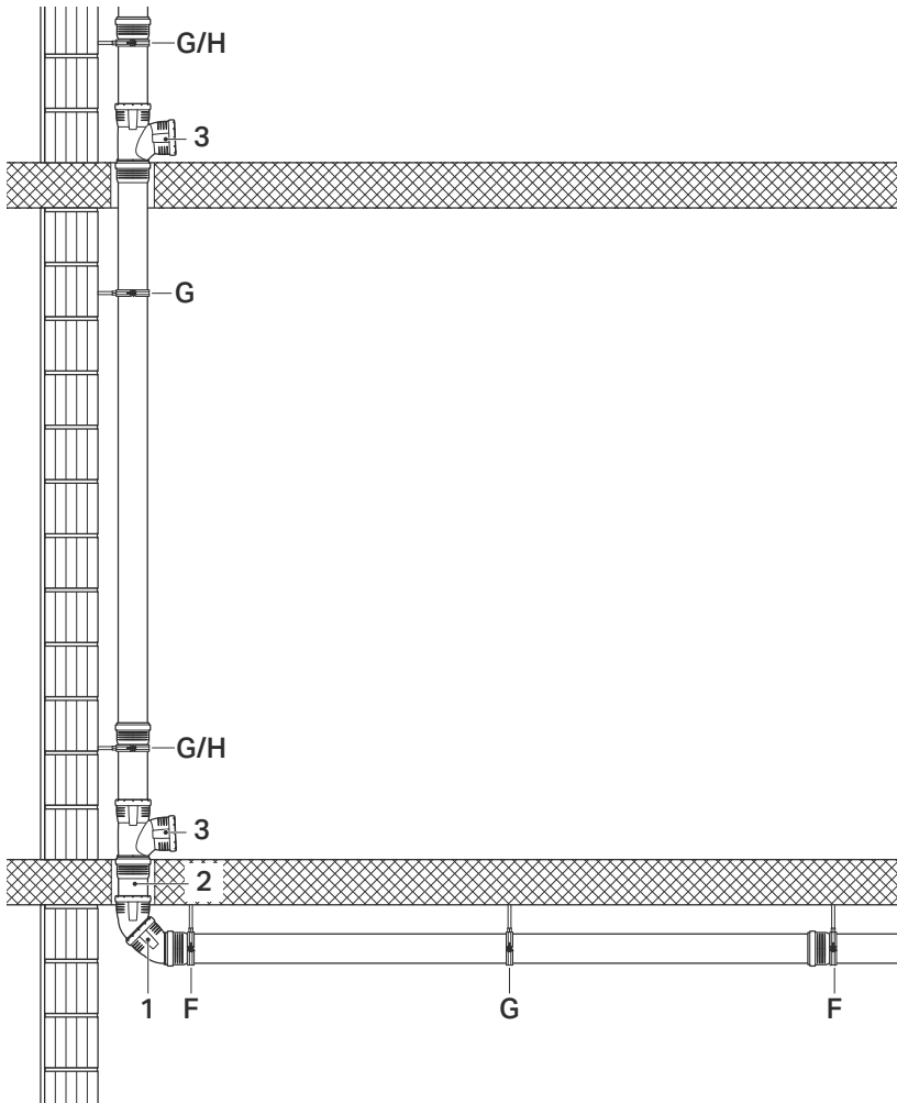
Abbildung 19: Umlenkung 2 x Bogen 45° mit Geberit Silent-Pro; Gleitschellen mit Haltefunktion in Bodennähe
