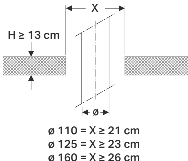
Abbildung 12: Aussparungsgrößen Geberit Mauerkragen (Ø 125 nicht für Geberit Silent-db20)
