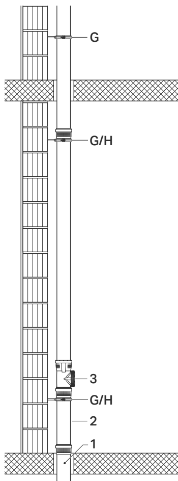
Abbildung 15: Fallleitung mit Geberit Silent-Pro
