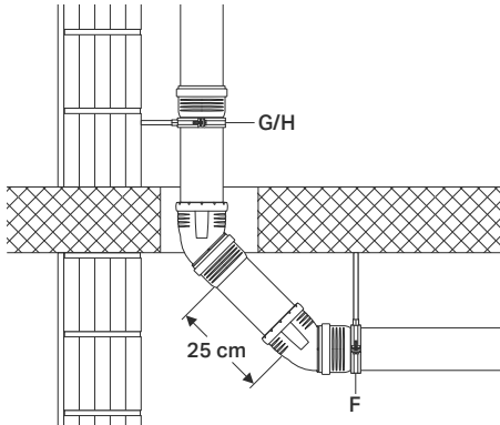
Abbildung 8: Beruhigungsstrecke bei Fallleitungsumlenkung
