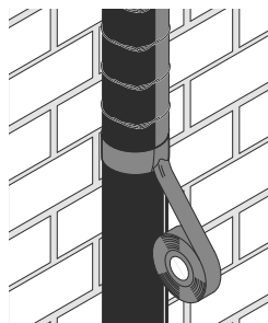
Abbildung 14: Schwitzwasserdämmung mit Geberit Schalldämmmatte Isol Flex
