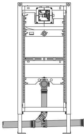
Abbildung 22: Anschlussmöglichkeit von Urinal-Abgang. Abgangsbogen mit Außendurchmesser 50 mm können direkt in Geberit Silent-Pro Steckmuffen eingesteckt werden.
