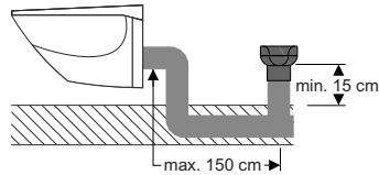
Abbildung 26: Geberit Belüftungsventil GRB90 an WC
