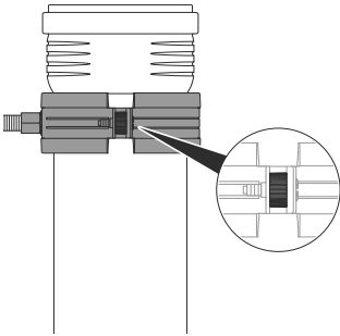
Abbildung 3: Gleitschelle mit Abstandhalter unterhalb der Steckmuffe
