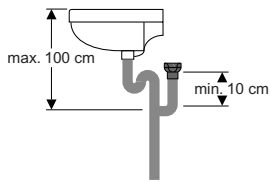
Abbildung 23: Geberit Belüftungsventil GRB50 an Waschbecken
