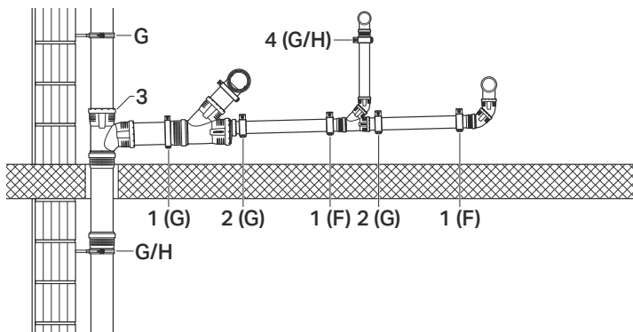
Abbildung 20: Sammelanschlussleitung mit Geberit Silent-Pro
