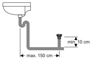
Abbildung 24: Geberit Belüftungsventil GRB50 an Waschbecken
