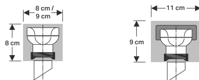
Abbildung 28: Maße für Geberit Belüftungsventil GRB50 ohne und mit Isolation
