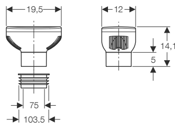
Abbildung 29: Maße für Geberit Belüftungsventil GRB90
