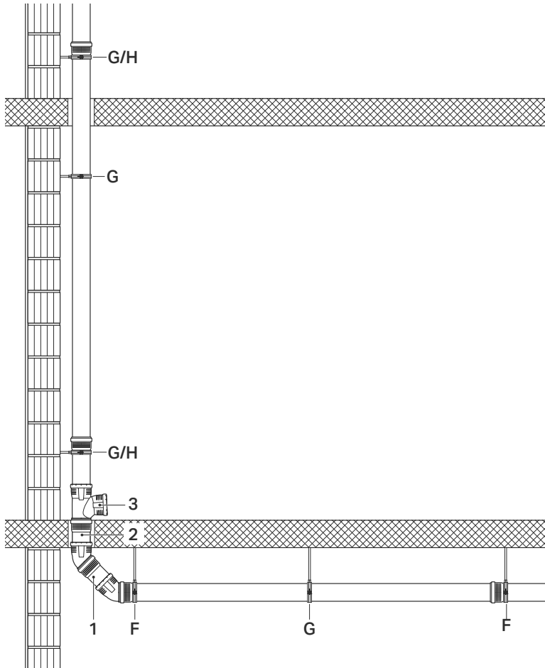
Abbildung 17: Umlenkung 2 x Bogen 45° und Beruhigungsstrecke mit Geberit Silent-Pro; Gleitschellen mit Haltefunktion in Bodennähe
