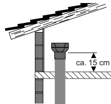
Abbildung 27: Geberit Belüftungsventil GRB90 unter Dach
