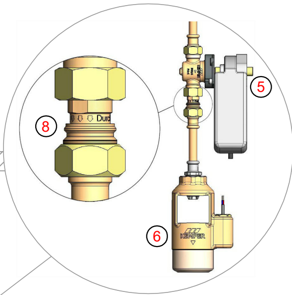
Durchflussmengenbegrenzer (DMB)
